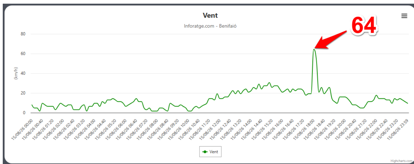
Ráfagas de viento máximas registradas en BENIFAIÓ el 15/08/26 (en km/h) https://inforatge.com/meteo-benifaio
